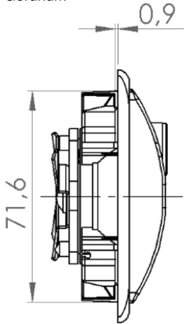
Yandan Görünüm
