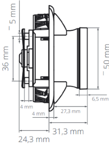
Yandan Görünüm
