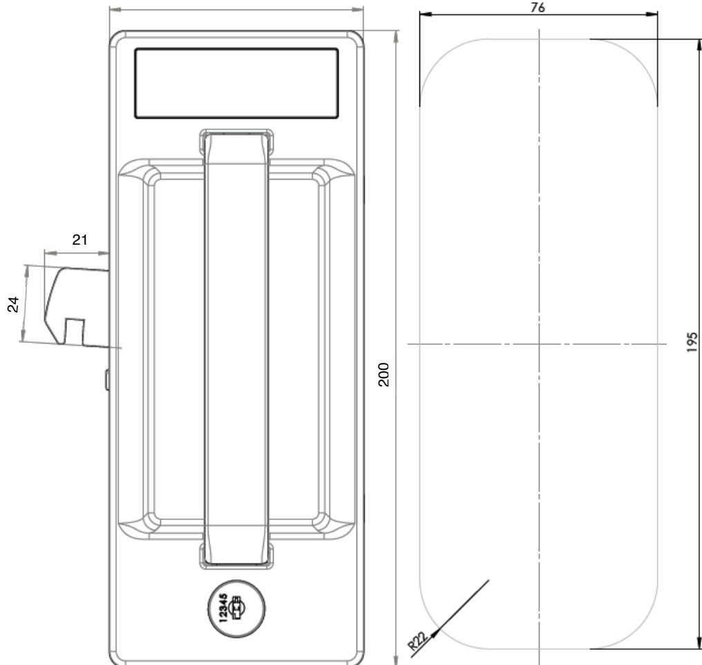
Ürün Ölçüleri
