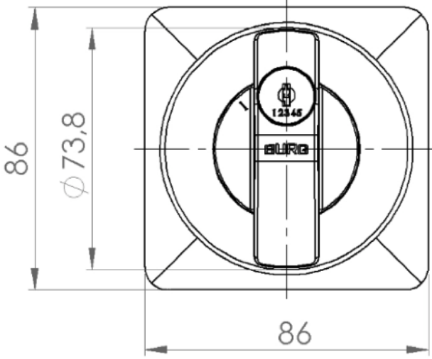
Önden Görünüm
