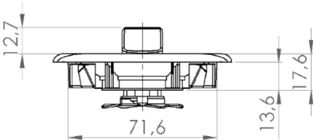
Üstten Görünüm
